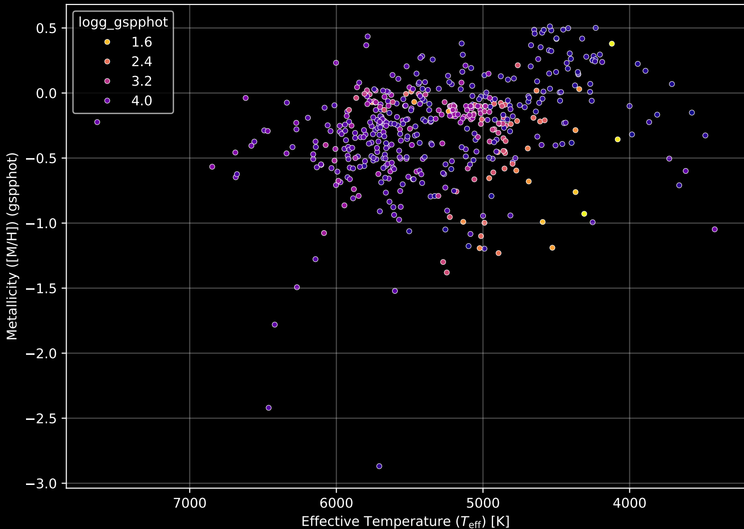
APOGEE DR17 Field: [VOD3] Stellar Population Parameters (n= 489)
